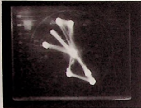
Bild 5: Vektor-Oszillogramm Kamera-Direktgang, Norm-Farbbalken bei Sonnenlicht
