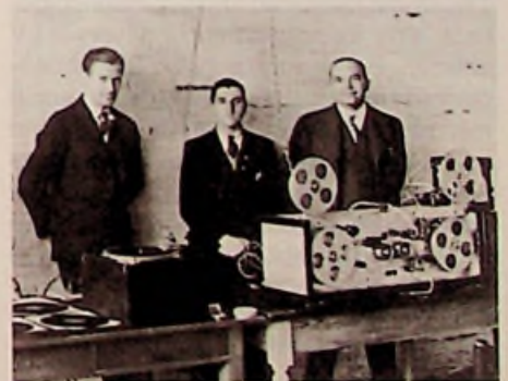
Bild 1: Das erste Magnetophon und sein Erfinder Eduard Schüller (links).
