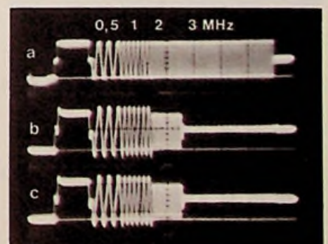
Bild 2: Video-Übertragungsbereich a) Multi-burst 0,5–4,8 MHz vor Band. b) über Band bei v_0 . c) über Band bei 0,5v_0
