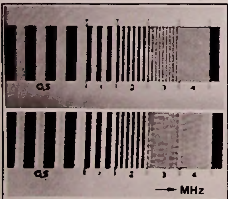
Bild 4: Horizontal-Auflösung a) Kamera-Direktgang b) nach Aufzeichnung und Wiedergabe (E etwa 2000 Lux)
